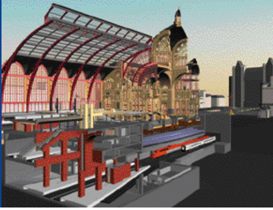
De spoortunnel onder Antwerpen-Centraal
